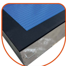
SOLIDE SCHWEISSKONSTRUKTION AUS 3-MM-BLECH, FEUERVERZINKT
