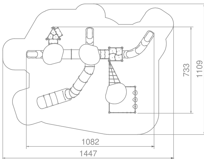
MASSSTAB 1:200
