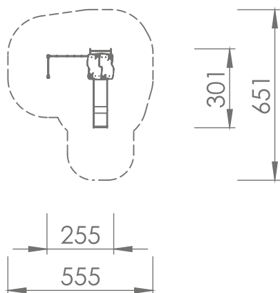
SCALE 1:120
