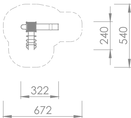
SCALE 1:120
